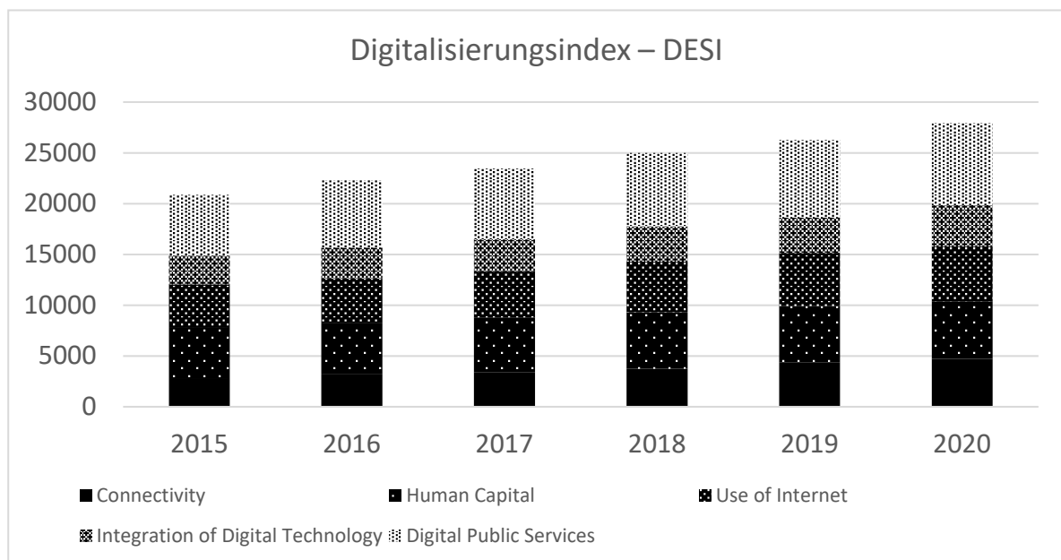
Abbildung 5: DESI-Index 2015 bis 2020
